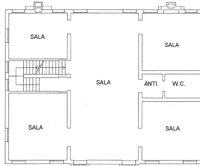
PIANTA PIANO PRIMO H= 360
